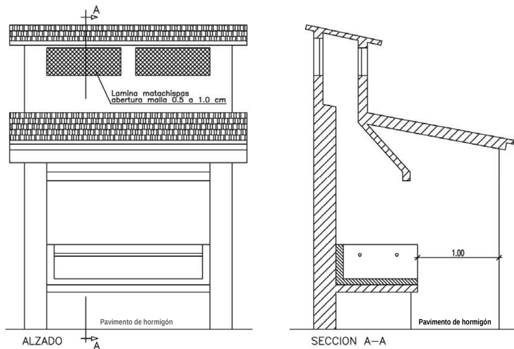
Imagen 1. Croquis de las dimensiones para construcción de un paellero autorizado para uso con fuego en el término municipal de Olocau.
